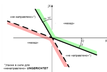
Рис. 6-31 Характеристика направления на R-X-плоскости
