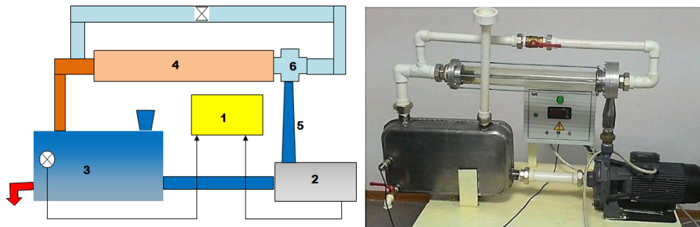
Рисунок 1 - Принципиальная схема (а) и фото (б) ВТГ: 1 - блок управления; 2 - гидравлический насос; 3 - бак с водой; 4 - вихревая труба; 5 - дроссель (сопло); 6 – завихритель
