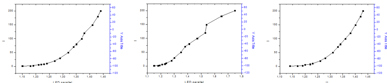
Рисунок 1. ВАХ светодиодов
