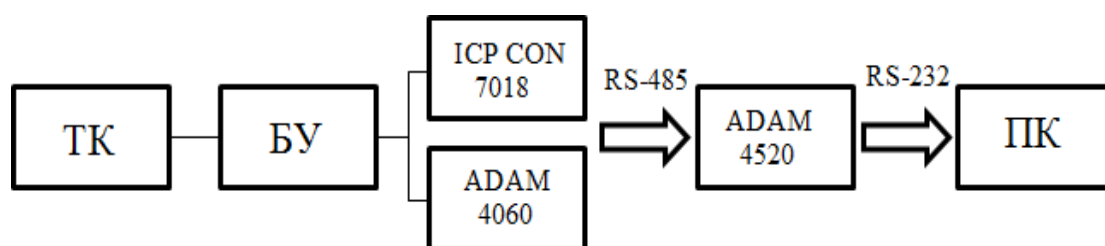
Рисунок 1.2 - Структурная схема подключения установки «Методы и технические средства измерения температуры ИВ1»
