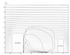
Рис.2. Распределение концентраций CO . Скорость ветра 8 м/с.
