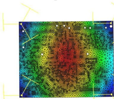
Рисунок 1 – Расчет собственных частот электронной платы
