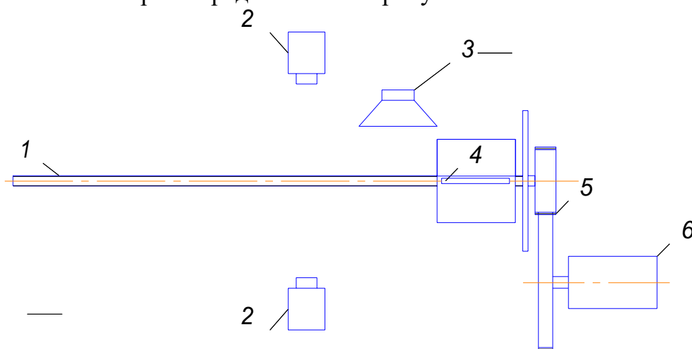
Рисунок 2 - Схема контроля
