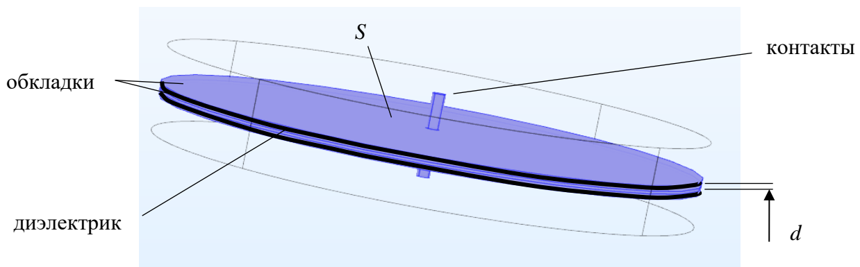
Рисунок 1 – Геометрия модели
