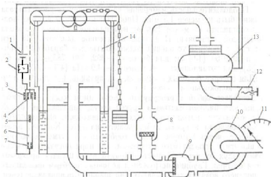
Рисунок 3 – Схема поверки газовых счетчиков с помощью источника электрического питания и датчика абсолютного давления: 1 – источник электрического питания; 2 – датчик абсолютного давления Метран-150ДА; 3-5, 7 – контакты; 6 – контактная линейка; 8-9 – клапаны; 10 – компрессор; 11 – регулируемая заслонка; 12 – выходная насадка; 13 – поверяемый счётчик; 13 – газовый мерник
