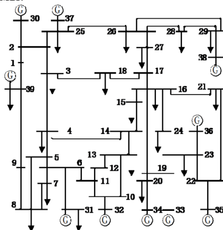
Рисунок 1 – Схема 39-шинной системы
