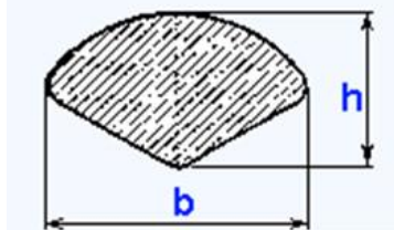
Рисунок 1 – Пример формы секторной жилы
