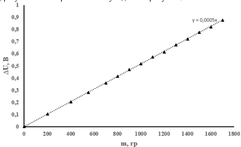
Рисунок 3 – Экспериментальная (♦) и теоретическая (.....) зависимости напряжения \Delta U разбаланса моста от массы ( m ) накладываемого на стальную пластину груза
