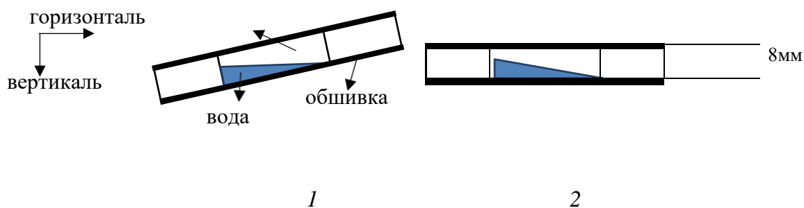
Рис. 1. Скопление воды в наклонной самолетной панели
