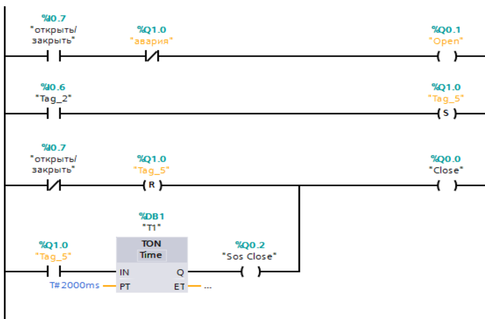
Рис. 4. Алгоритм открытия дверей на языке FBD
