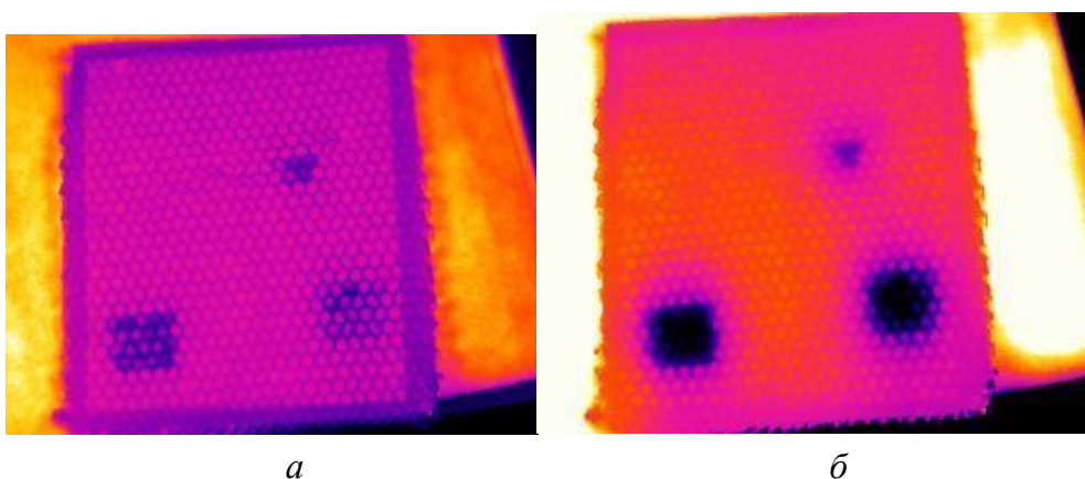
Рис. 2. Термограммы горизонтально расположенного образца: а – во время нагрева; б – через 10 с после нагрева
