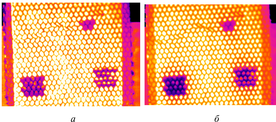
Рис. 1. Термограммы вертикально расположенного образца: а – 4 с после начала нагрева; б – 2 с после окончания нагрева
