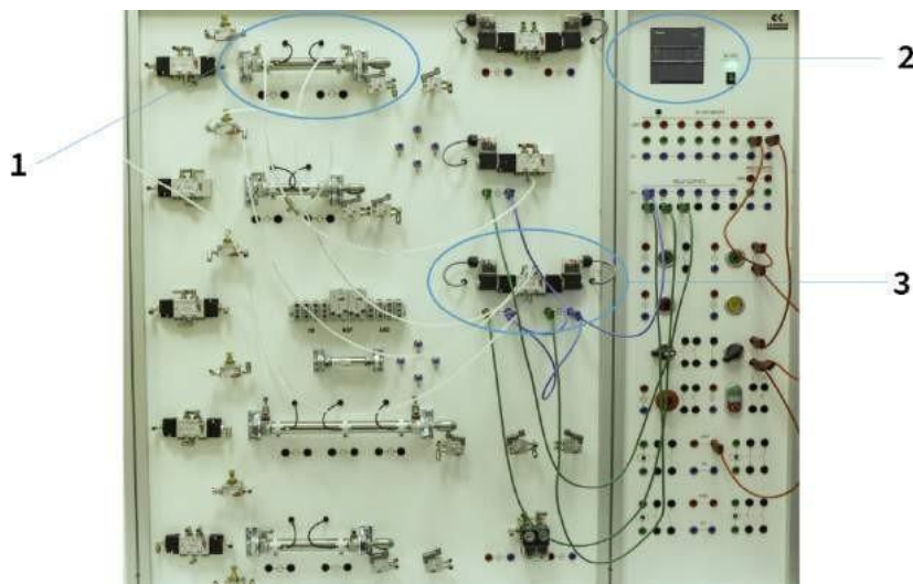
Рис.3. Стенд открытия дверей:
