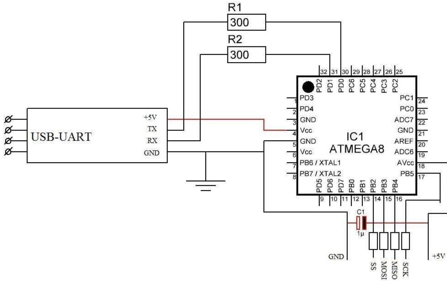
Рис. 1. Принципиальная схема преобразователя USB-SPI
