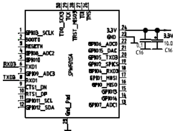
Рис. 3. Wi-Fi модуль
