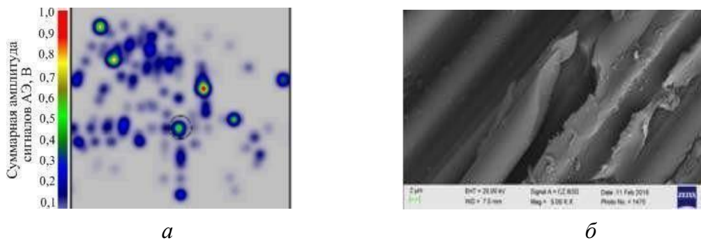
Рис. 3. Локация сигналов АЭ при нагружении образца до P = 35 кН (а) и результаты его фрактографии в области отверстия (б)
