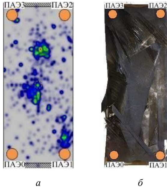
Рис. 2. Локация сигналов АЭ при разрушении образца (а); вид разрушенного образца (б)
