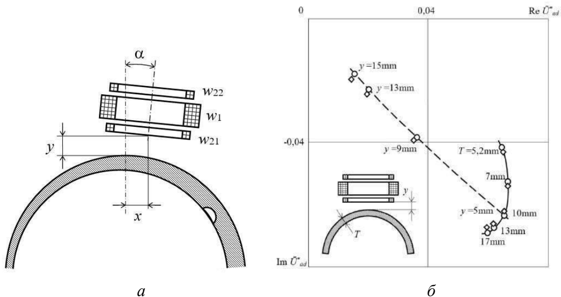
Рис. 1. Накладной ВТП, находящийся во взаимодействии с электропроводящей трубой (а) и расчетные (○) и экспериментальные (◇) зависимости относительного вносимого напряжения ВТП от изменения толщины стенки трубы T и зазора y (б)
