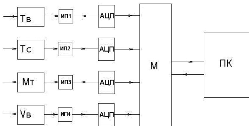
Рис. 4. Структурная схема контролируемых параметров: T_{в} – термометр влажный; T_{с} – термометр сухой; M_{т} – датчик для оценки влажности древесины; V_{в} – скорость воздушного агента; ИП – измерительный преобразователь; АЦП – аналого-цифровой преобразователь; М – микропроцессор; ПК – персональный компьютер
