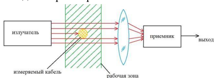
Рис. 1 - Метод измерения мощности потока излучения.
