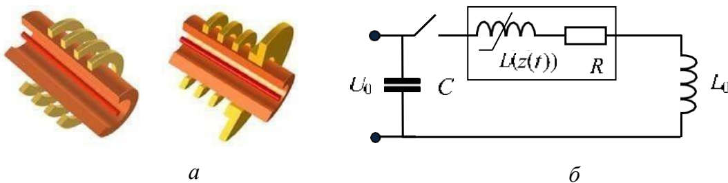
Рис. 1. Упрощенные модели КМПУ, отличающиеся емкостью и формой соленоида: а – сечение плазменного ускорителя; б – схема замещения
