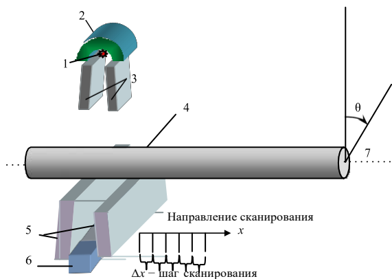
Рис. 1. Непрерывное (дискретное) вращение с дискретным линейным перемещением: 1 – источник излучения; 2 – радиационная защита источника; 3 – целевой коллиматор источника; ОК; 5 – целевой коллиматор детектора; 6 – линейка детекторов; 7 – ось вращения ОК
