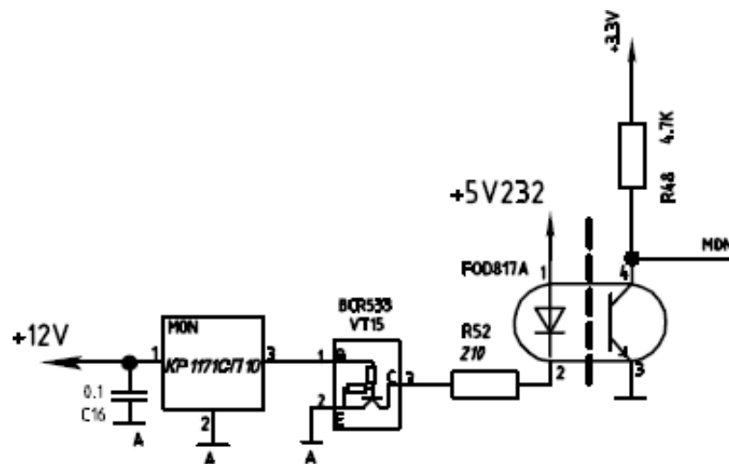
Рис. 5. Монитор питания
