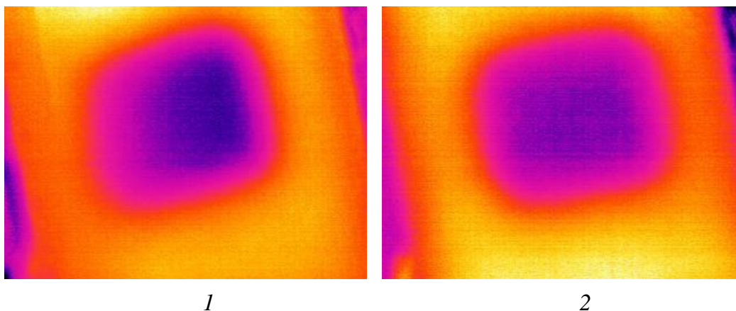
Рис. 4. Термограммы при стимуляции снизу: 1 – горизонтальная панель; 2 – наклонная панель (40 с)
