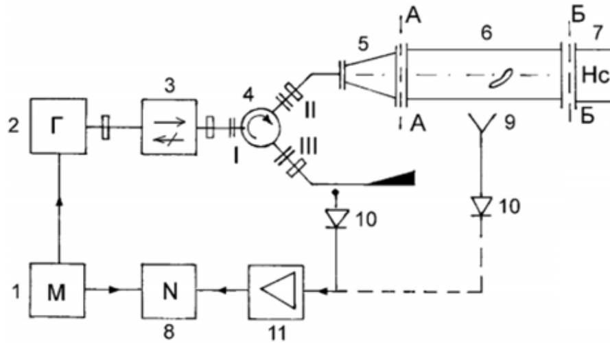
Рис. 1. Структурная схема лабораторного макета радиоволнового дефектоскопа: 1 – модулятор; 2 – СВЧ-генератор; 3 – вентиль; 4 – циркулятор; 5 – трансформатор типа волны; 6 – трубопровод; 7 – согласованная нагрузка; 8 – скоростной осциллограф; 9 – приемная антенна; 10 – СВЧ-детектор; 11 – усилитель
