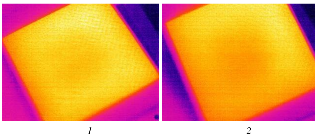
Рис. 5. Термограммы при стимуляции сверху: 1 – горизонтальная панель (100 с); 2 – наклонная панель (100 с)
