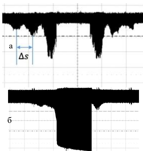
Рис. 2. Дифракционная картина полученная многоэлементным приёмником: а – с непрозрачным барьером, б – без непрозрачного барьера.
