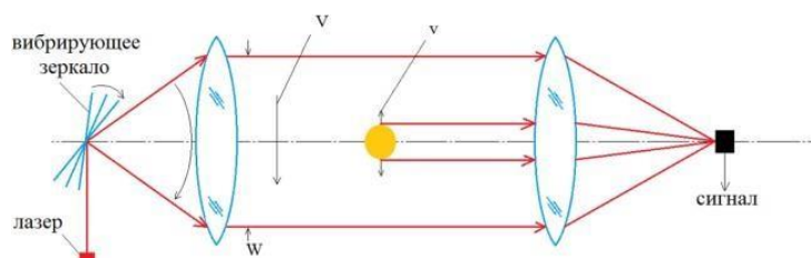
Рис. 2 - Схема со сканирующим узлом.
