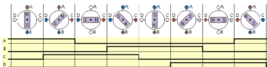
Рис. 3. Положения ротора в полушаговом режиме
