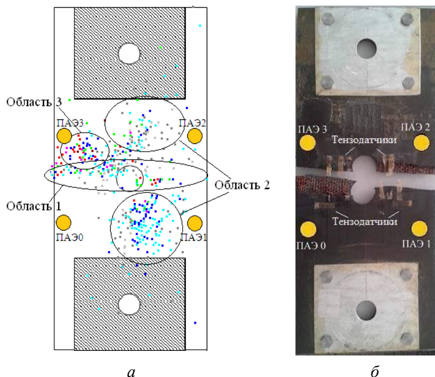
Рис.1. Локация сигналов АЭ, зарегистрированных в процессе нагружения образца 1 (а); внешний вид образца после разрушения (б)
