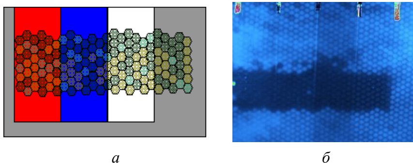
Рис. 3. Примерный вид дефектной области панели (а) и термограмма этой области (б)
