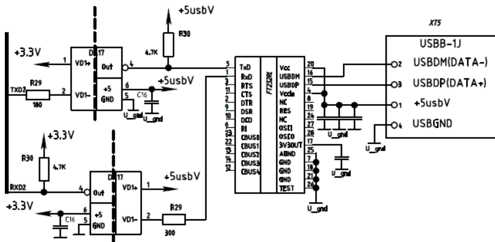
Рис. 7. USB-интерфейс
