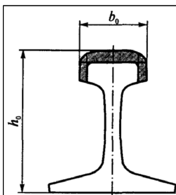
Рис. 1. Схематическое изображение бокового и вертикального износа h_0
