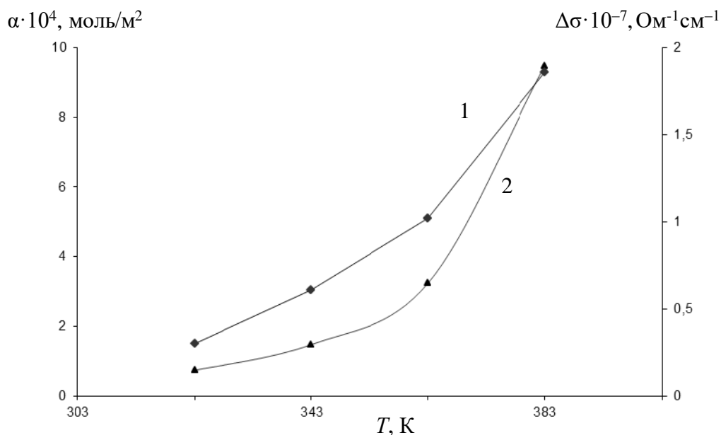
Рис. 1. Температурные зависимости изменения поверхностной электропроводности (1) и величины адсорбции (2) для образца 0,95\text{InSb}-0,05\text{ZnTe} в атмосфере \text{NH}_3 ( p = 5,3 \text{ Па} ).
