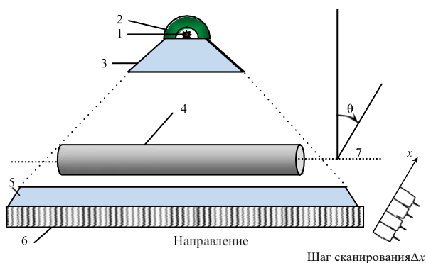
Рис. 3. Непрерывное (дискретное) линейное перемещение с дискретным вращением с формированием одномерных проекций: 1 – источник излучения; 2 – радиационная защита источника; 3 – коллиматор источника; 4 – ОК; 5 – коллиматор детектора; 6 – линейка детекторов; 7 – ось вращения ОК
